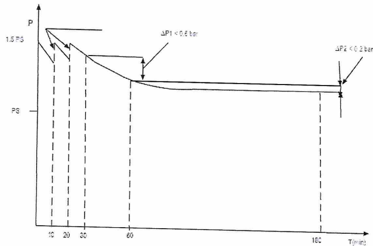
Figure 10 : Essai d'étanchéité
